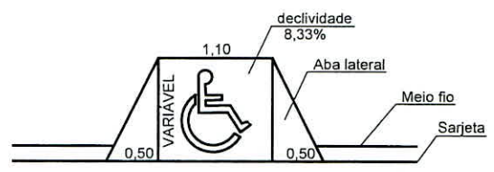
Detalhe - Rampa p/ portadores de deficiência motora
