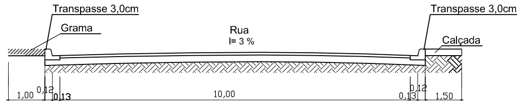
PERFIL TRANSVERSAL DA RUA
